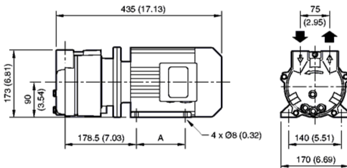
Габаритные размеры
