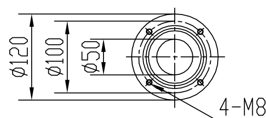
Фланец входной
