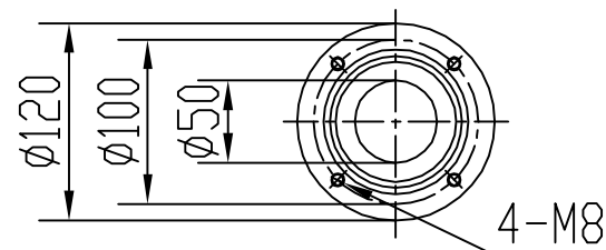
Фланец выходной
